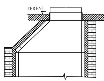
PRIEREZ A-A
