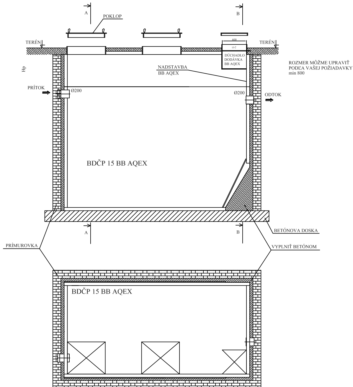
PRIEREZ A-A
