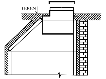
PRIEREZ B-B
